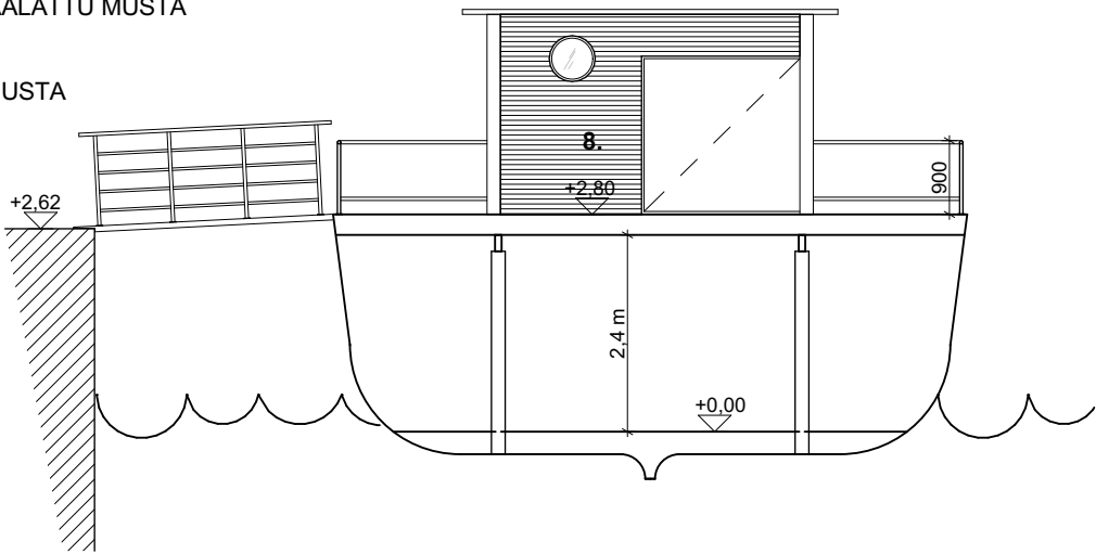
LEIKKAUS A-A
